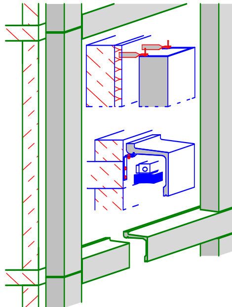
Prinzipdarstellung
